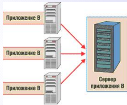
Рисунок 2.8: Консолидация приложений
