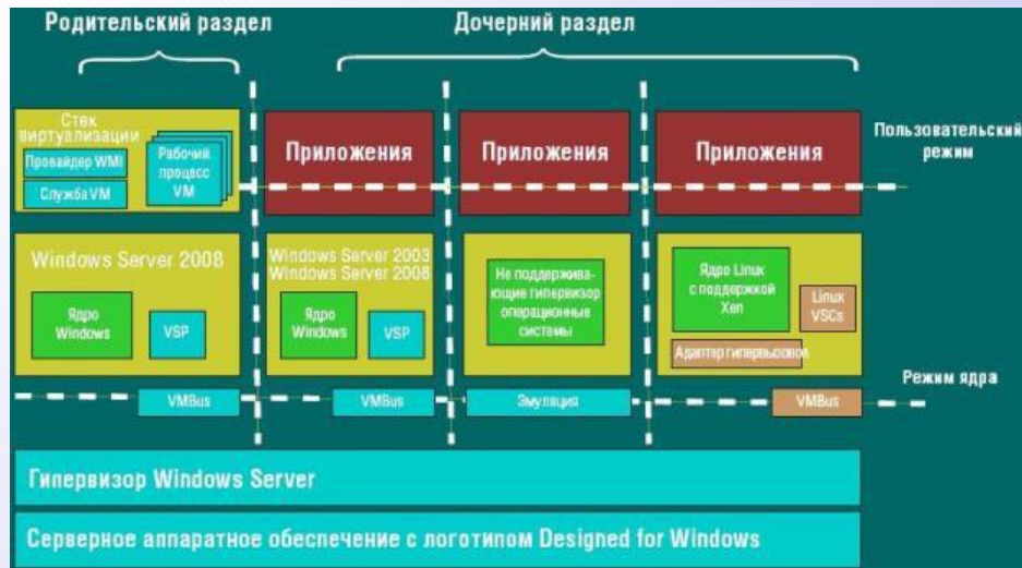
Рисунок 3.15: Архитектура Hyper-V
