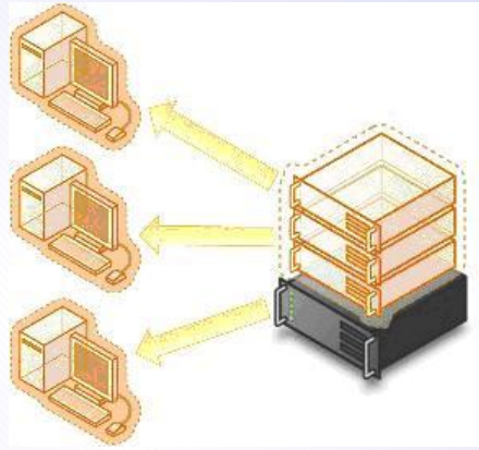
Рисунок 3.8: Виртуализация представлений
