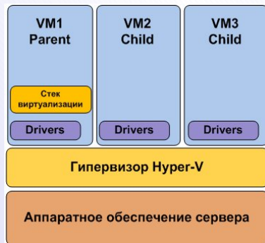
Рисунок 3.14: Архитектура микроядерного гипервизора
