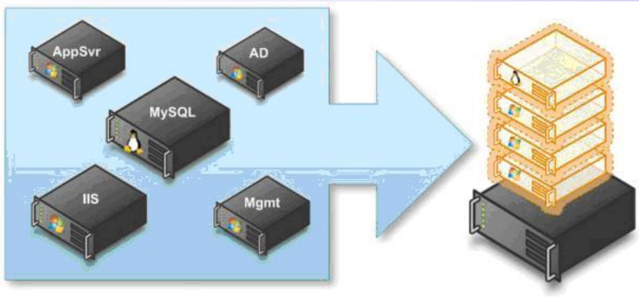
Рисунок 3.3: Виртуализация серверов
