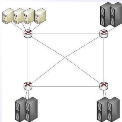
Рисунок 2.6: Структура Решетка
