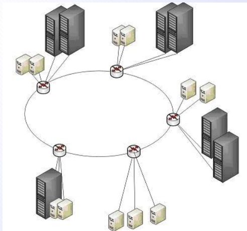
Рисунок 2.7: Структура Кольцо
