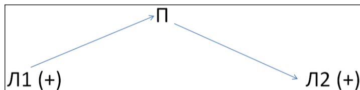
Рисунок 6. – Положительная минимальная ЛП-система
