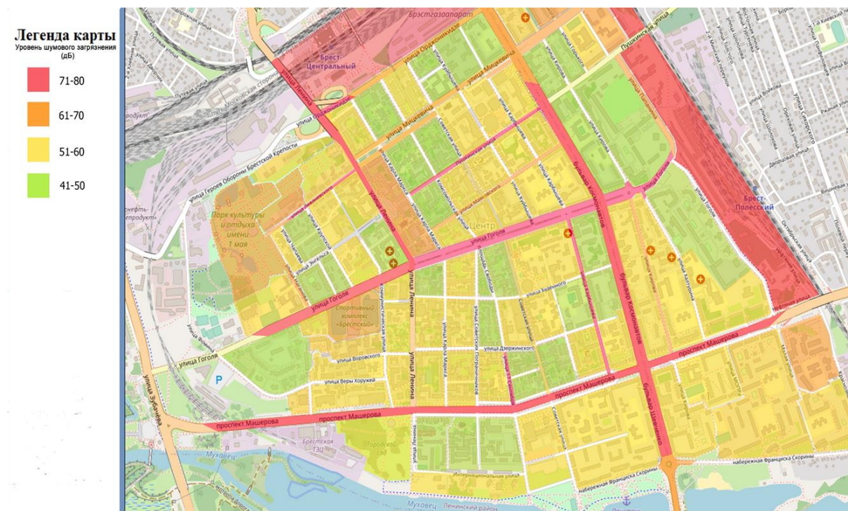
Рисунок 1 – Карта шумового загрязнения микрорайона «Центр»
