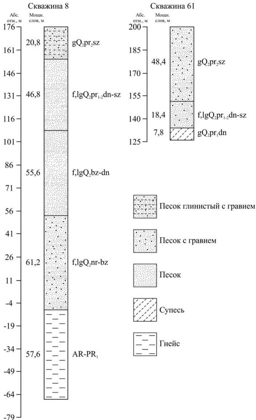
Рисунок 2 – Стратиграфические колонки скв. 8 и 61, характеризующие строение четвертичных отложений в районе расположения месторождения песчано-гравийных пород «Козловичи»
