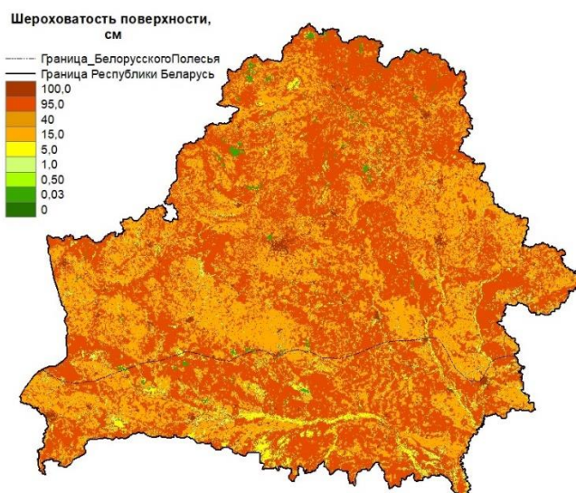
Рисунок 2 – Параметр шероховатости подстилающей земной поверхности для территории Беларуси
