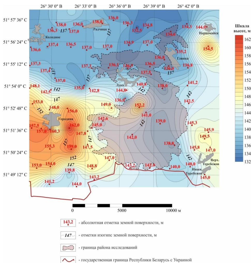
Рисунок 2 – Гипсометрическая схема восточной части болотного массива Морочно и прилегающих территорий
