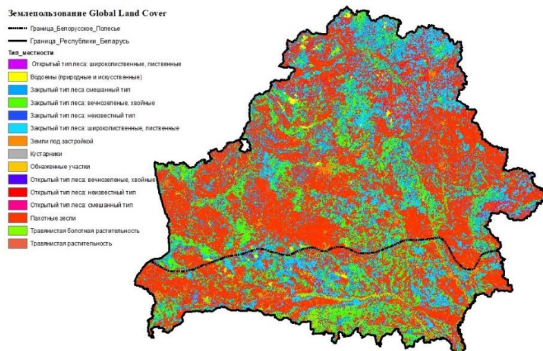
Рисунок 1 – Классификация типов земной поверхности для территории Беларуси
