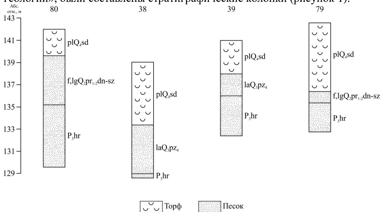
Рисунок 1 – Стратиграфические колонки скв. 80, 38, 39 и 79, характеризующие строение покровных отложений территории восточной части болотного массива Морочно
