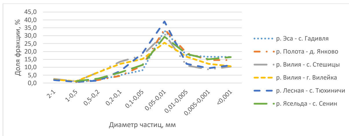
Рисунок – Осредненные значения гранулометрического состава взвешенных наносов для исследуемых рек
