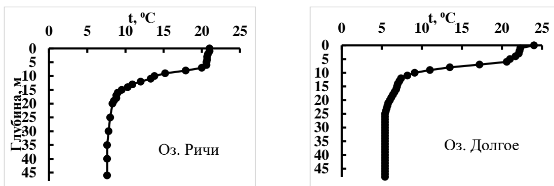
Рисунок 1 – Распределение температуры (°C) по глубине
