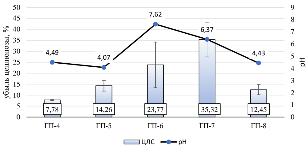
Рисунок 1 – Интенсивность разложения целлюлозы
