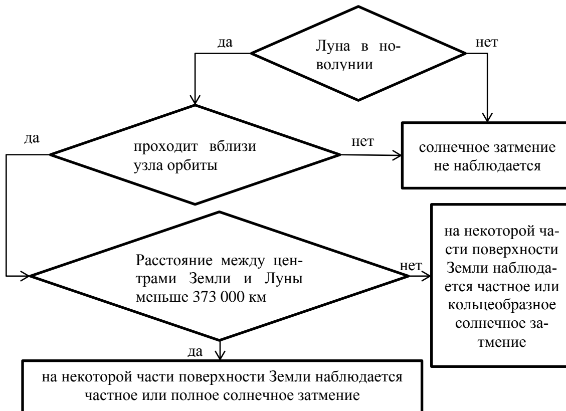
Рисунок – Блок-схема алгоритма определения возможности наблюдения солнечного затмения
