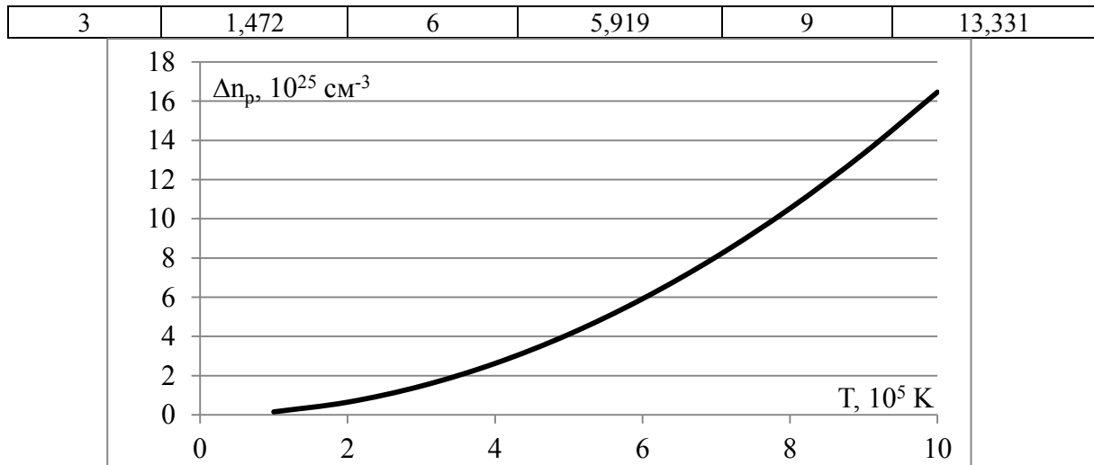
Рисунок 1. – Значение \Delta n_p , соответствующее порогу нейтронизации при различных температурах, согласно уравнению (24)
