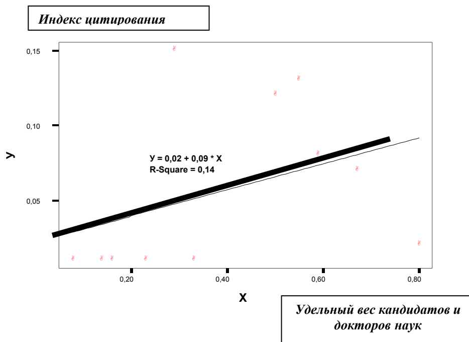
Рисунок 2 – Регрессионная модель y = 0,09x + 0,02
