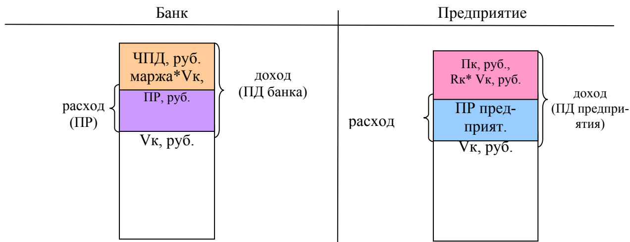
Рисунок 3 – Чистый процентный доход банка и предприятия от кредитования
