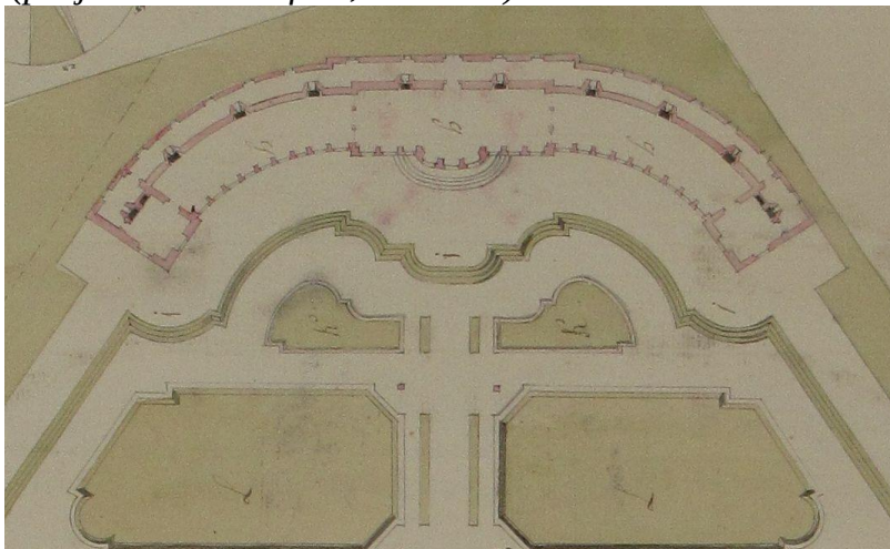
II. 9. Ołyka-Turczyn. Projekt oranżerii. Fragm. projektu ogrodu Na Turczynie (proj. J. G. Knackfuss; ok. 1752). Fot. ze zbiorów autora
