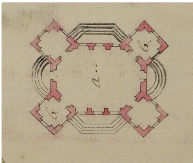
II. 6. Ołyka-Turczyn. Projekt pawilonu molino da vento . Fragm. projektu ogrodu Na Turczynie (proj. J. G. Knackfuss; ok. 1752). Fot. Ze zbiorów autora
