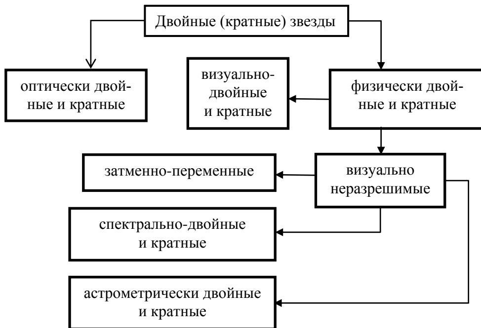
Рисунок – Классификация двойных и кратных звезд
