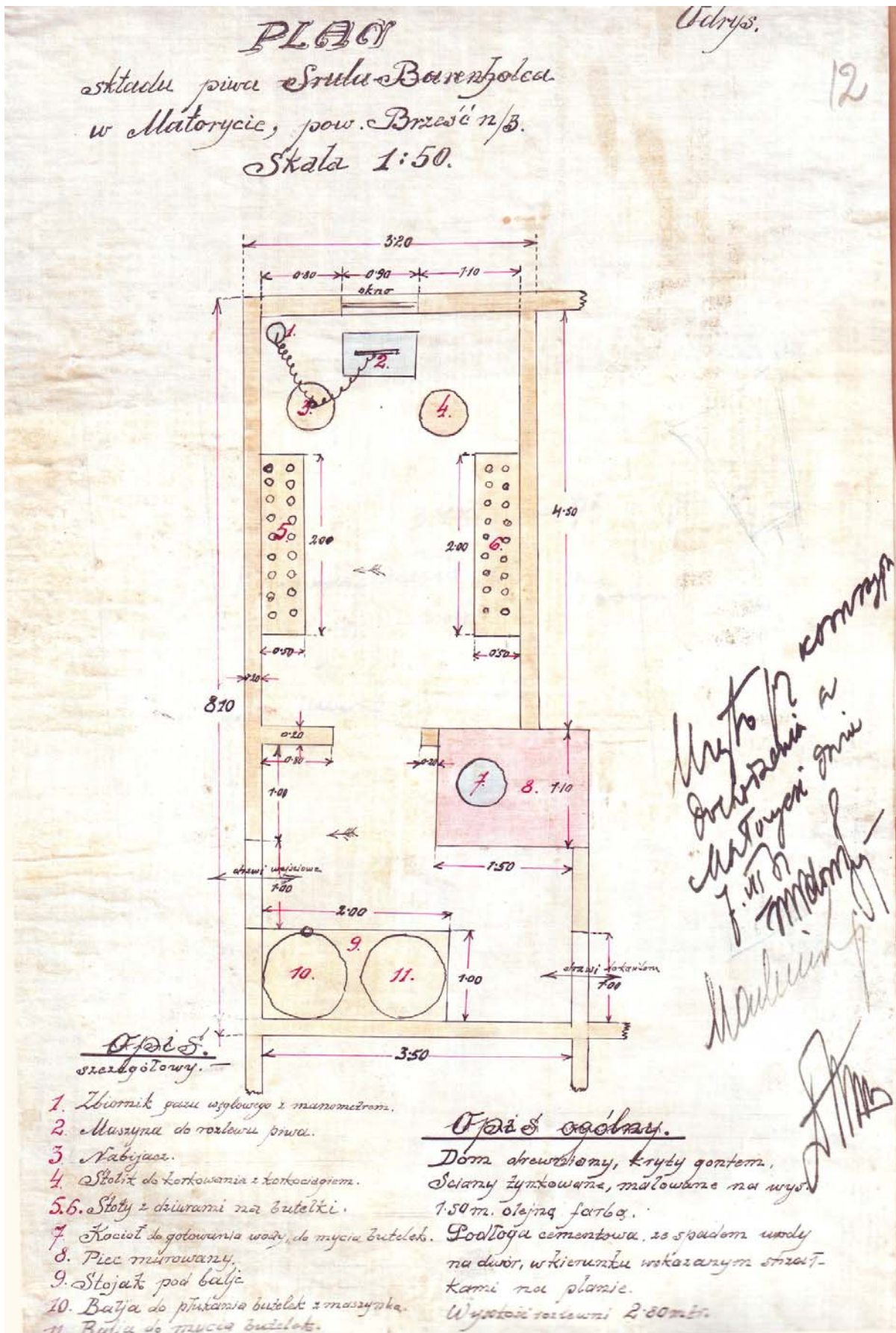
Рисунок 2. – План разливочной
