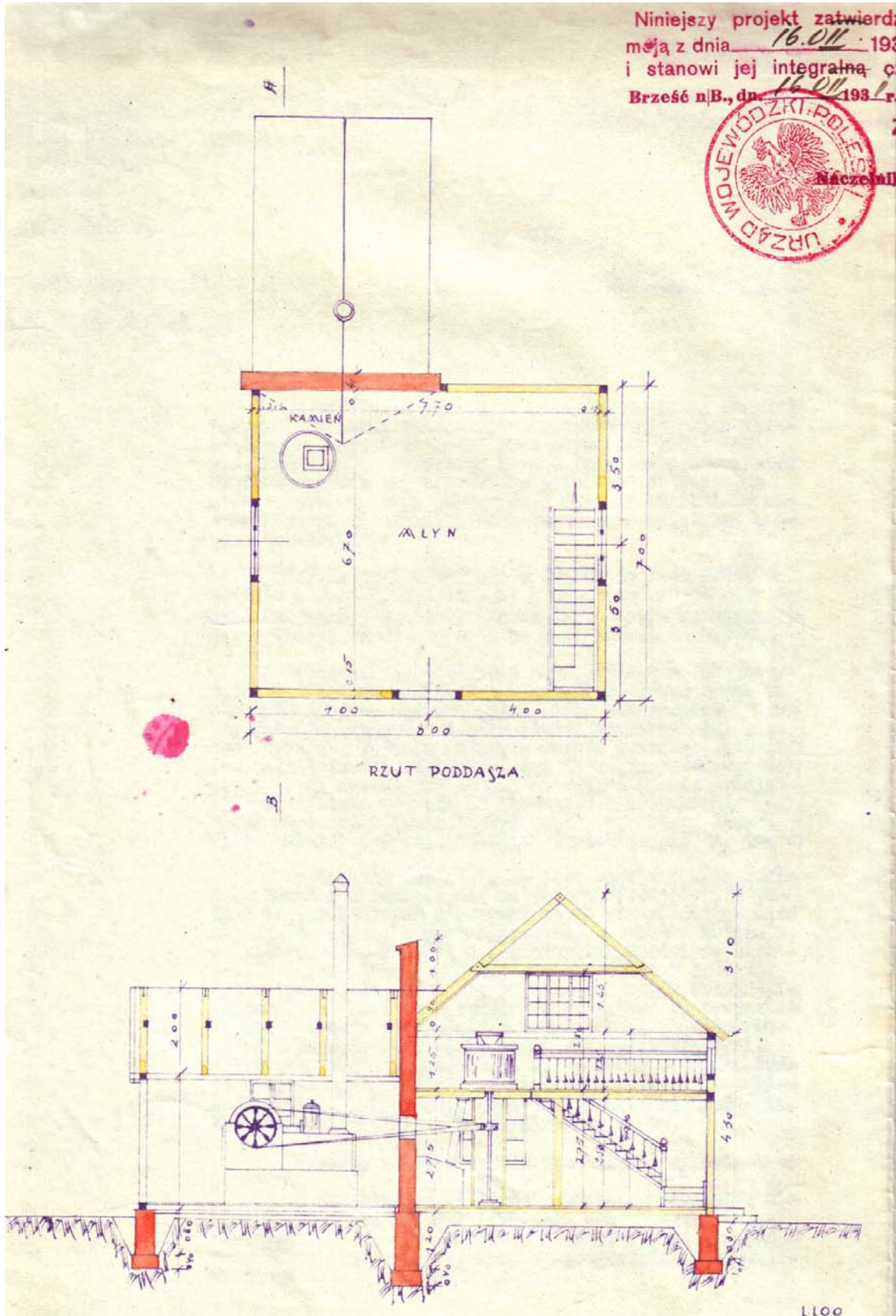
Рисунок 1. – План мельницы
