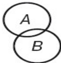
Рисунок 2 – Перекрещивающиеся понятия
